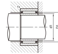
保持器軸向定位 由軸承箱孔側面
