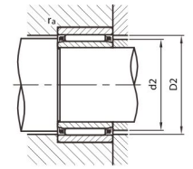
保持器軸向定位 由軸肩側面
