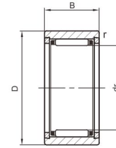
NK ,NKS ( dr \leq 10\text{mm} )
