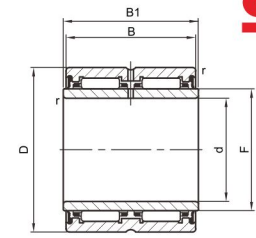
RNA69...2RS(F≥40)
