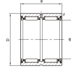
NA69...2RS(F≥40)
