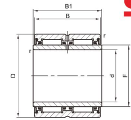
RNA69...2RS(F≥40)
