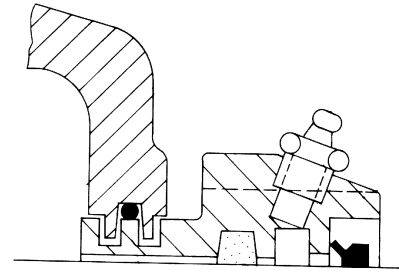
Optional taconite seal TER/ Joint d'étanchéité en taconite TER optionnel
